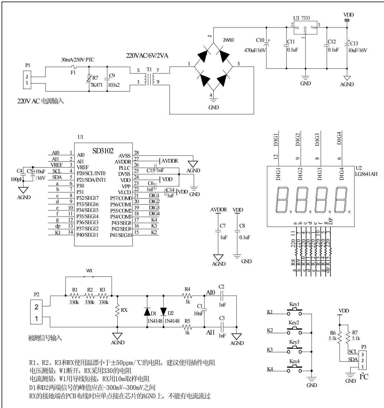
图 4.2 单相交、直流电压或电流测量（数码管显示）典型应用图
