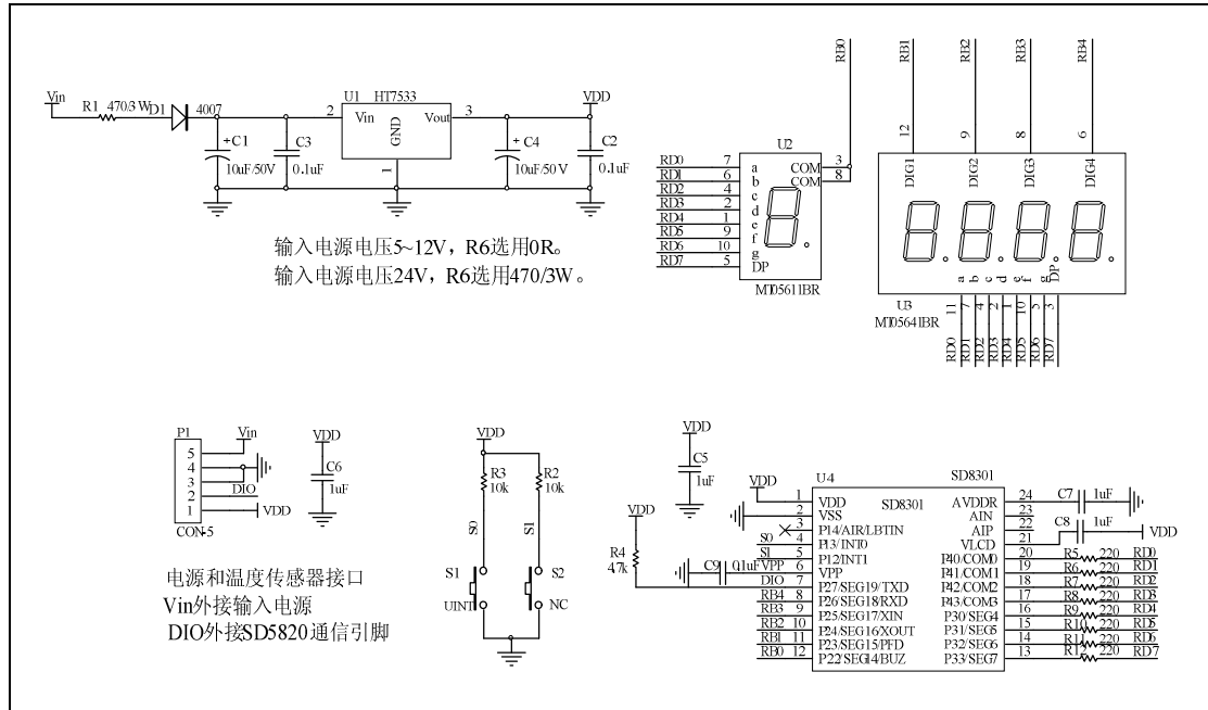
图2 电路原理图
