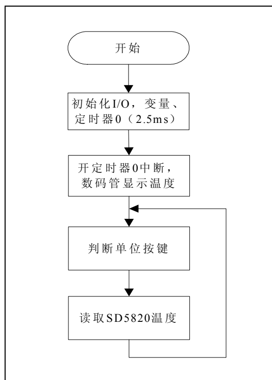
图3 程序流程图
