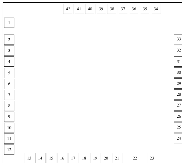
图1. PAD 图
