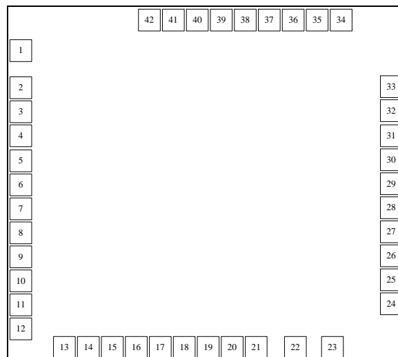
图 1. PAD 图
