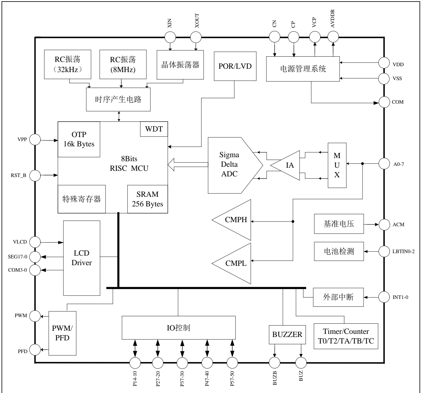
图2. 功能框图
