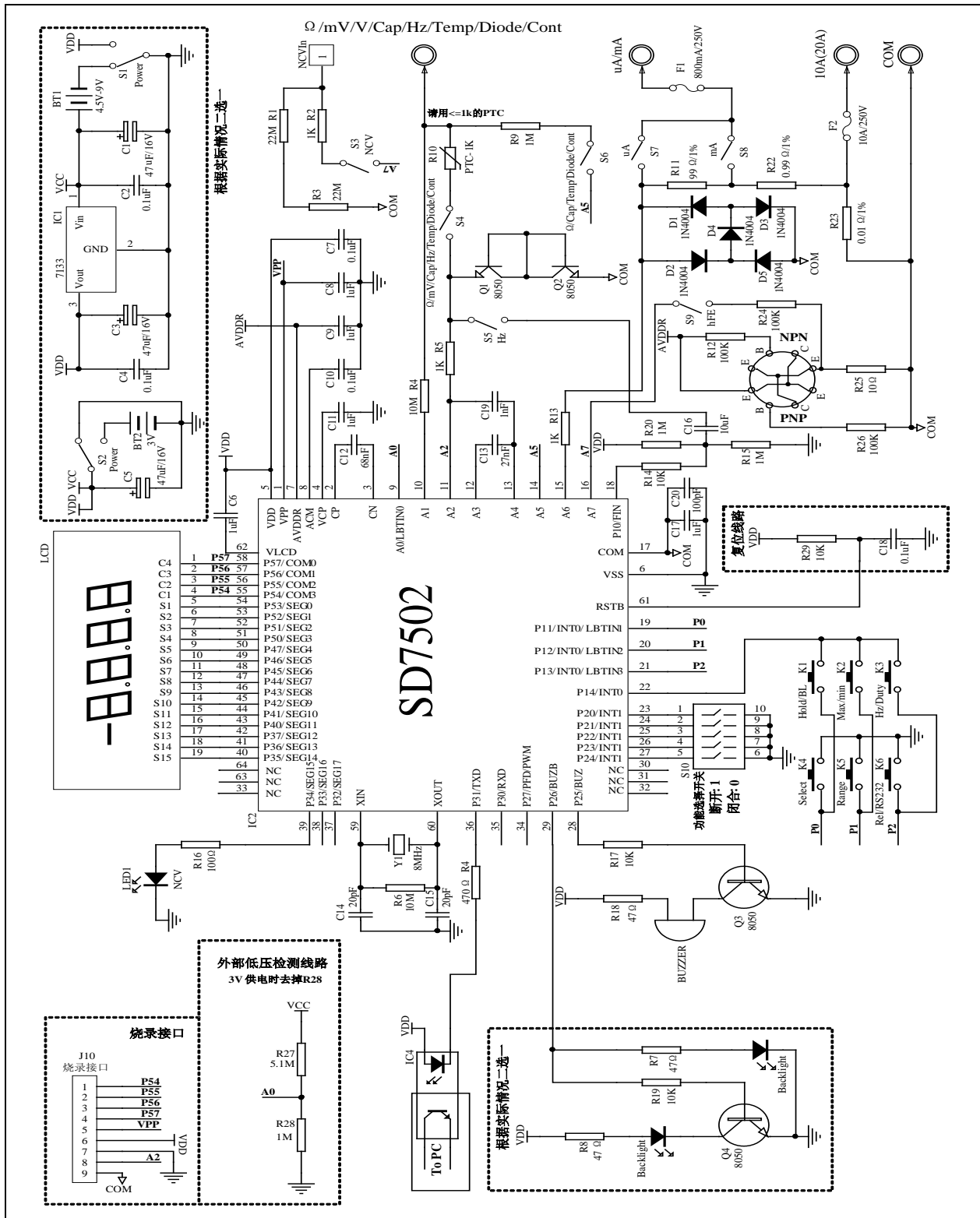
图3. 典型应用图
