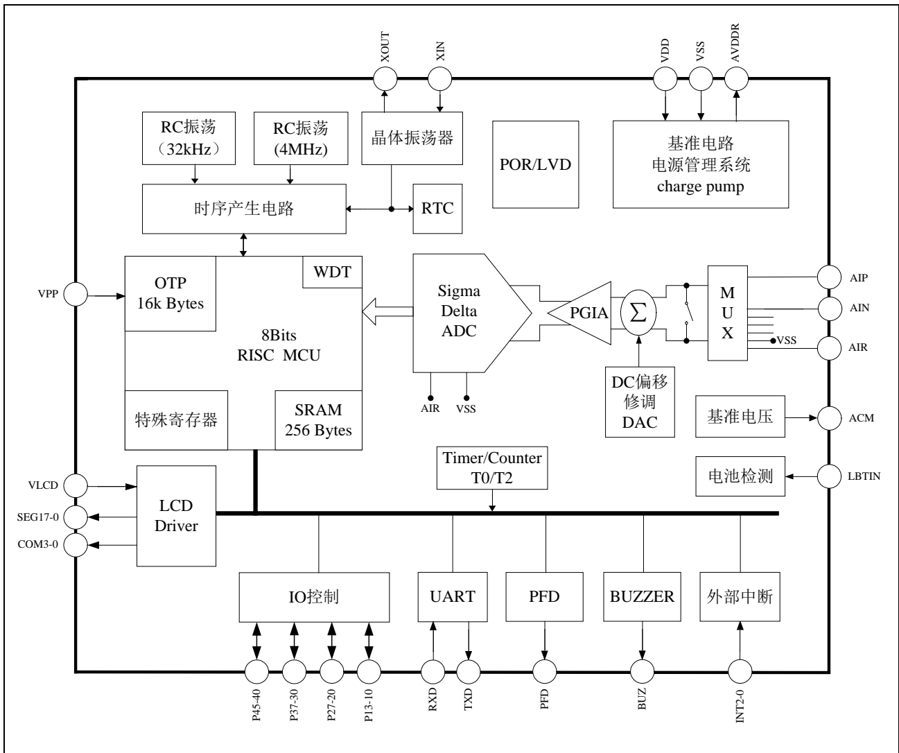
图2. 功能框图
