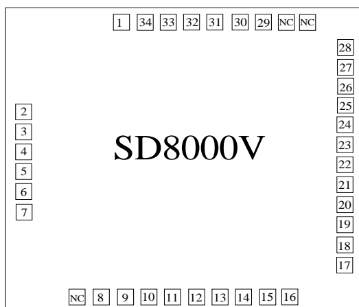
图 1. PAD 图
