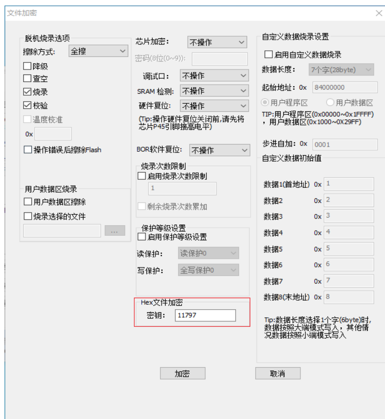
图 4.18.2 文件加密
