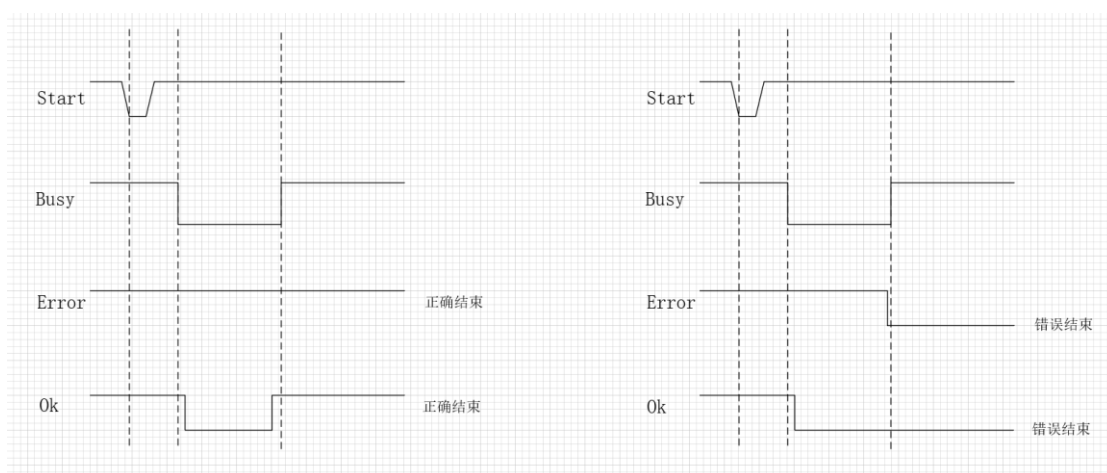
图 5.1 烧录器对接烧录机信号时序图
