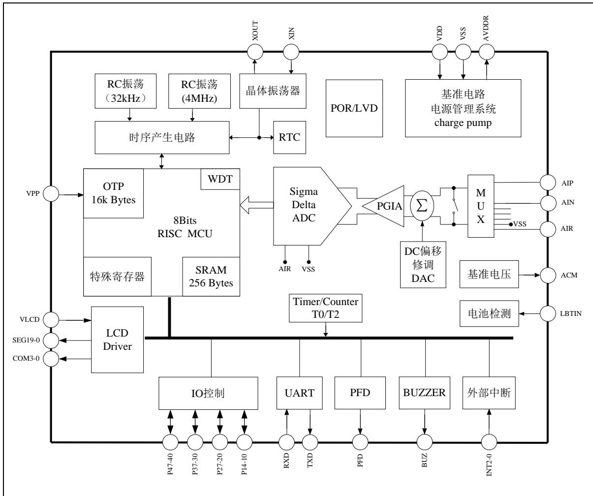
图2. 功能框图
