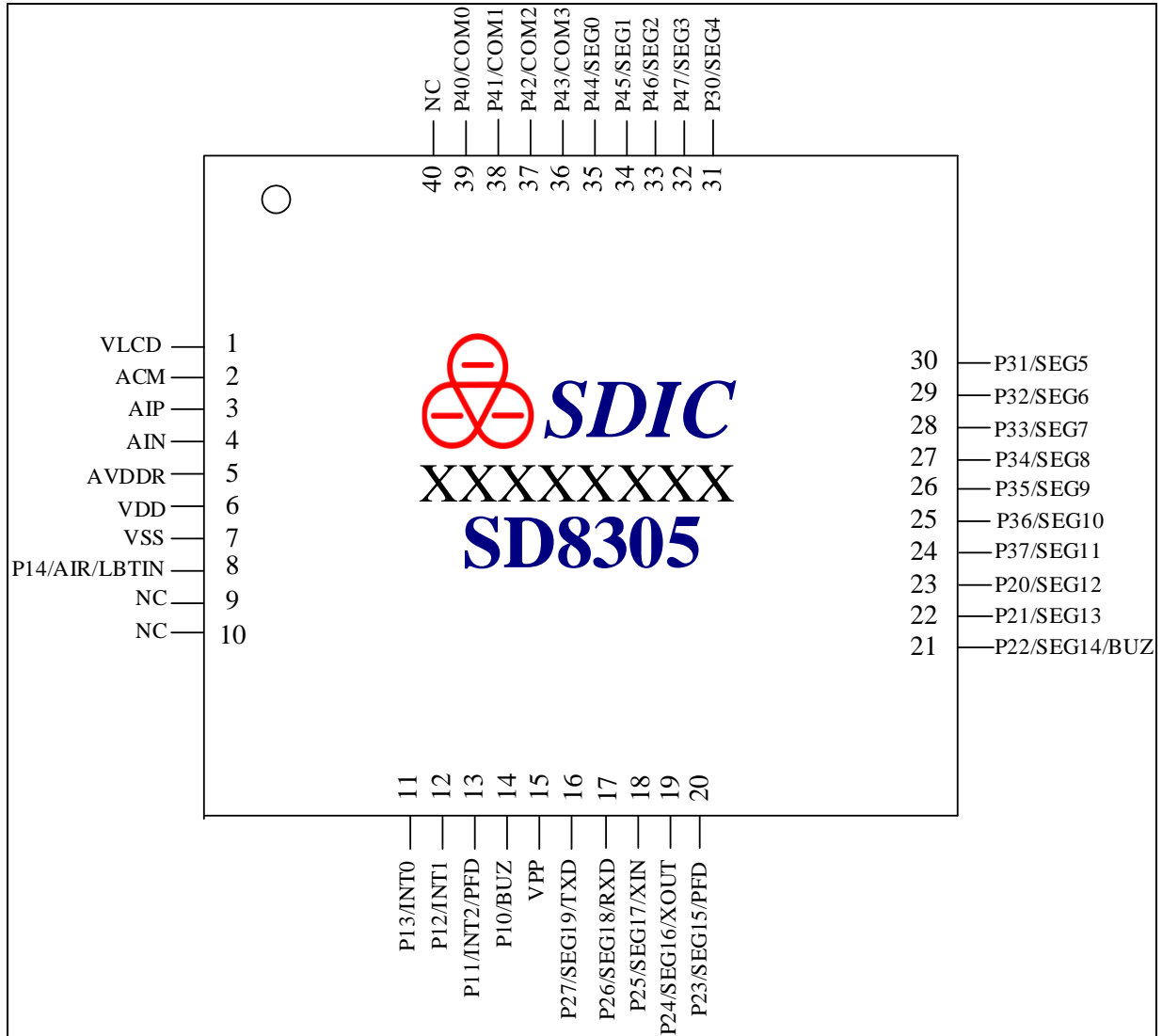
图1. 管脚图
